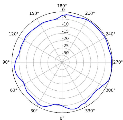
5GHz (Horizontal)
