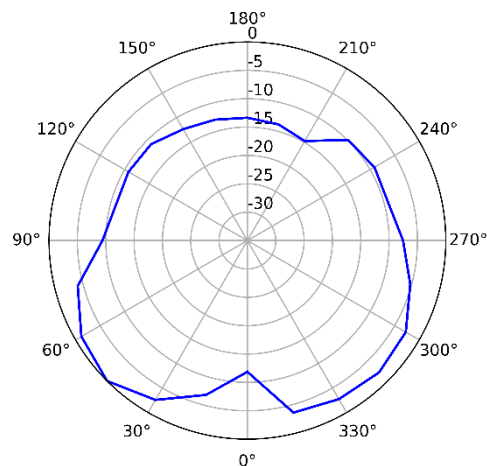
5GHz (Vertical)
