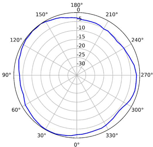
5GHz(Horizontal)
