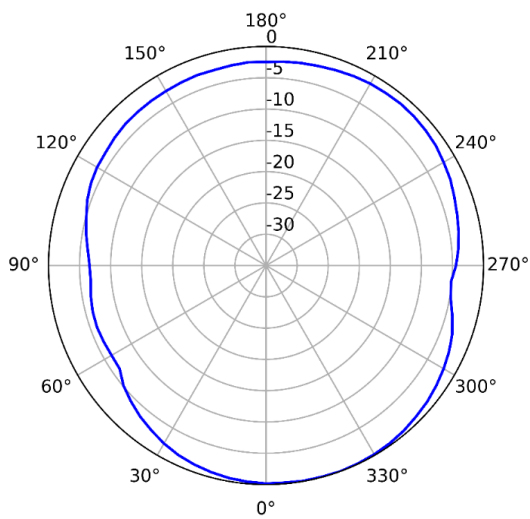
2.4GHz(Horizontal)
