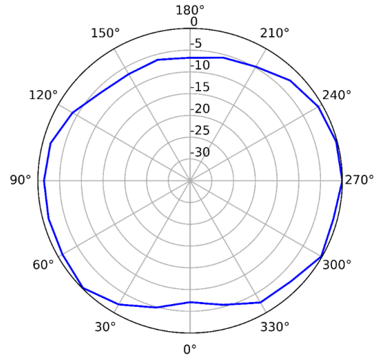
5GHz(Vertical)
